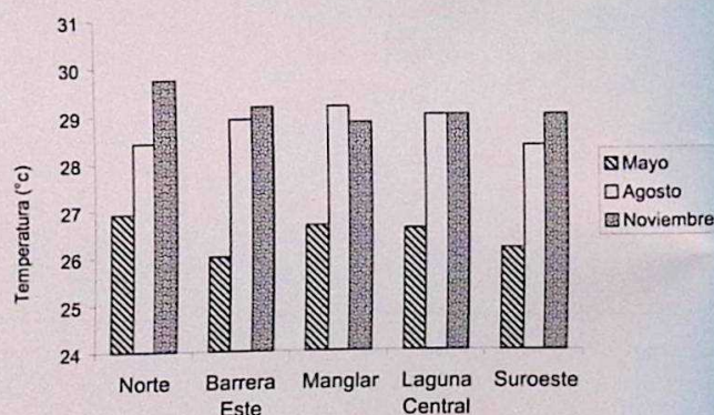
Fig. 3. Variación de la temperatura superficial del agua en las zonas Norte; Barrera Este; Manglar; Laguna Central y Suroeste, durante los meses de mayo, agosto y noviembre del año 2000.
