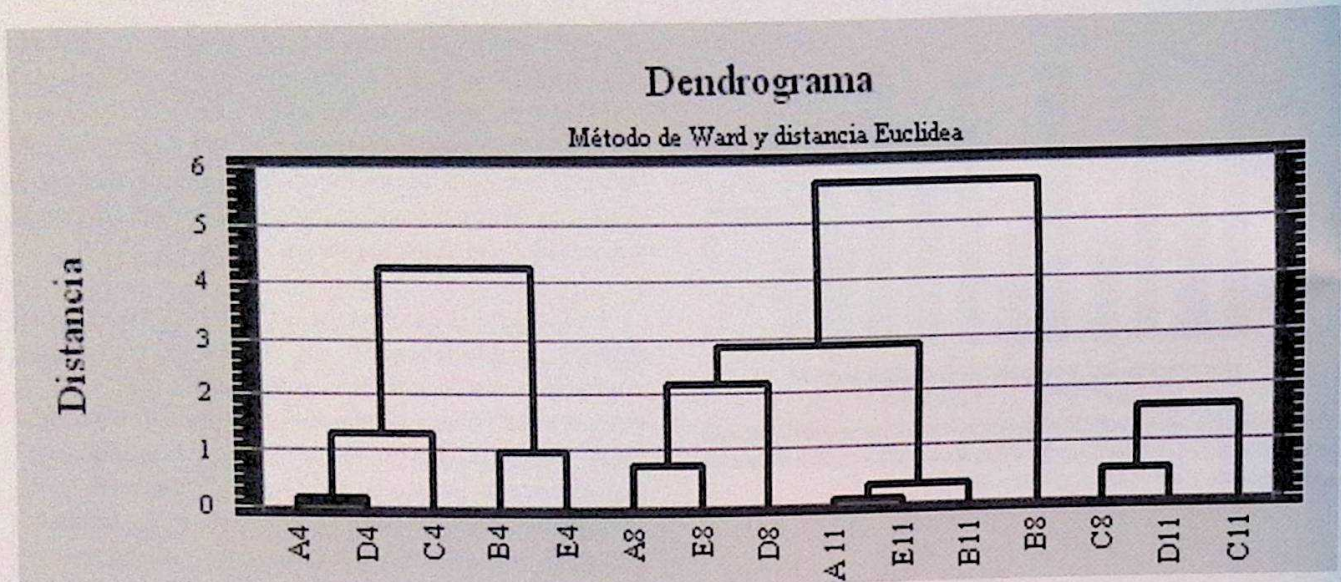
Fig. 6. Dendrograma vertical de los parámetros fisicoquímicos en función de las zonas (A: Norte; B: Barrera Este; C: Manglar; D: Laguna Central; E: Suroeste) y meses (4: mayo; 8: agosto; 11: noviembre).
