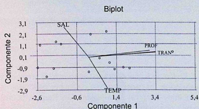
Fig. 5. Análisis de Componentes Principales de los parámetros fisicoquímicos evaluados en las zonas estudiadas durante los meses de mayo, agosto y noviembre.
