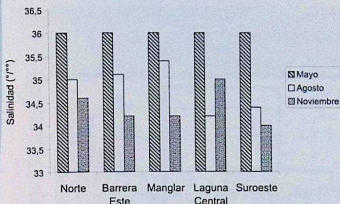
Fig. 4. Variación de la salinidad del agua en las zonas Norte; Barrera Este; Manglar; Laguna Central y Suroeste, durante los meses de mayo, agosto y noviembre del año 2000.
