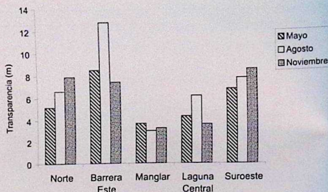
Fig. 2. Variación de la transparencia del agua en las zonas de estudio, durante los meses de mayo, agosto y noviembre del año 2000
