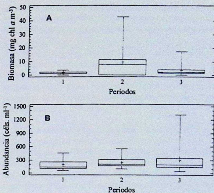
Fig. 4. Variación estacional de la biomasa fitoplanctónica (concentración de clorofila a , A, y abundancia fitoplanctónica, B) en playa San Luis, Cumaná, Venezuela. 1= Período de Calma; 2= Período de Surgencia y 3= Período de Transición.
