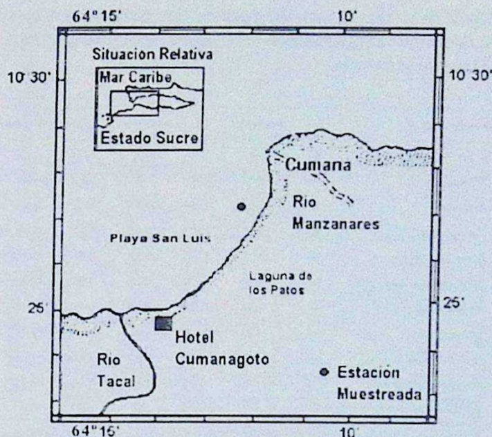
Fig. 1. Área de estudio mostrando la ubicación de la estación objeto de estudio.
