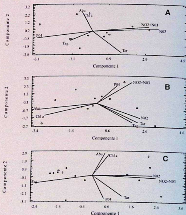
Fig. 5. Proyección ortogonal de algunas variables físico-químicas y biológicas medidas en la playa San Luis (Cumaná) en el espacio definido por los primeros dos componentes del ACP para los periodos de: calma, A; surgencia, B; transición, C.
