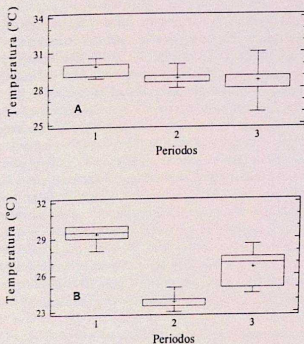
Fig. 2. Variación estacional de la temperatura del aire (A) y del agua (B) en la playa San Luis, Cumaná, Venezuela. 1= Período de Calma; 2= Período de Surgencia y 3= Período de Transición.
