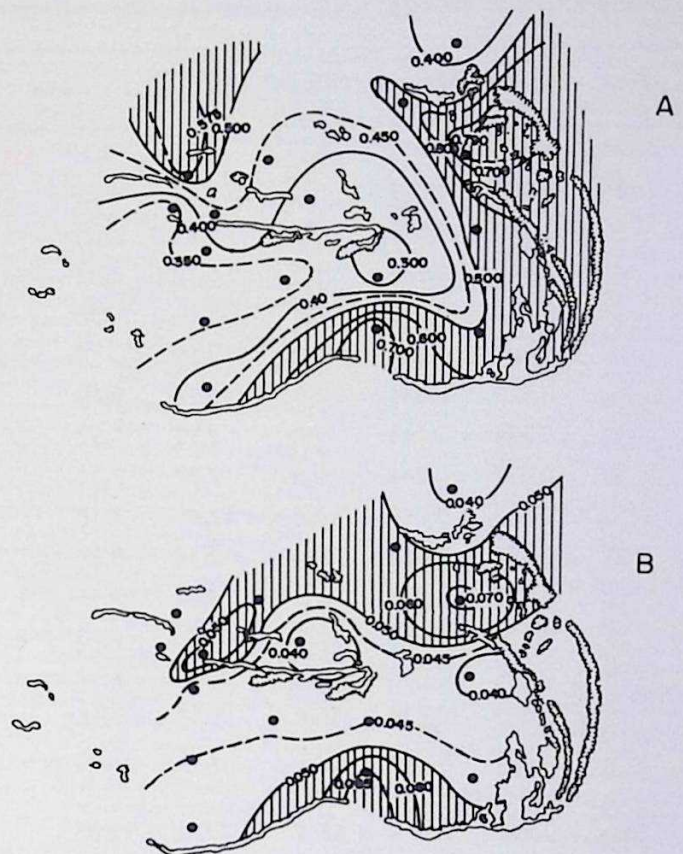
Figura 2.- Distribución espacial (A y B) del contenido de C-org. (%) y N-org. (%) en los sedimentos del Archipiélago Los Roques.
