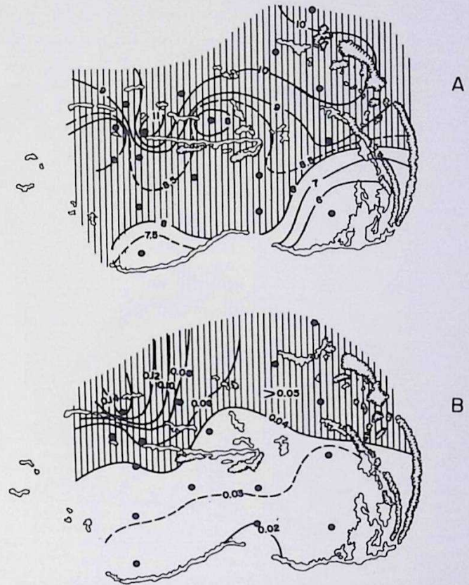
Figura 4.- Variación estacional (A y B) de las concentraciones de nitrógeno total (N-total %) y de ortofosfatos ( \text{P}_2\text{O}_5 %) en los sedimentos del Archipiélago Los Roques.
