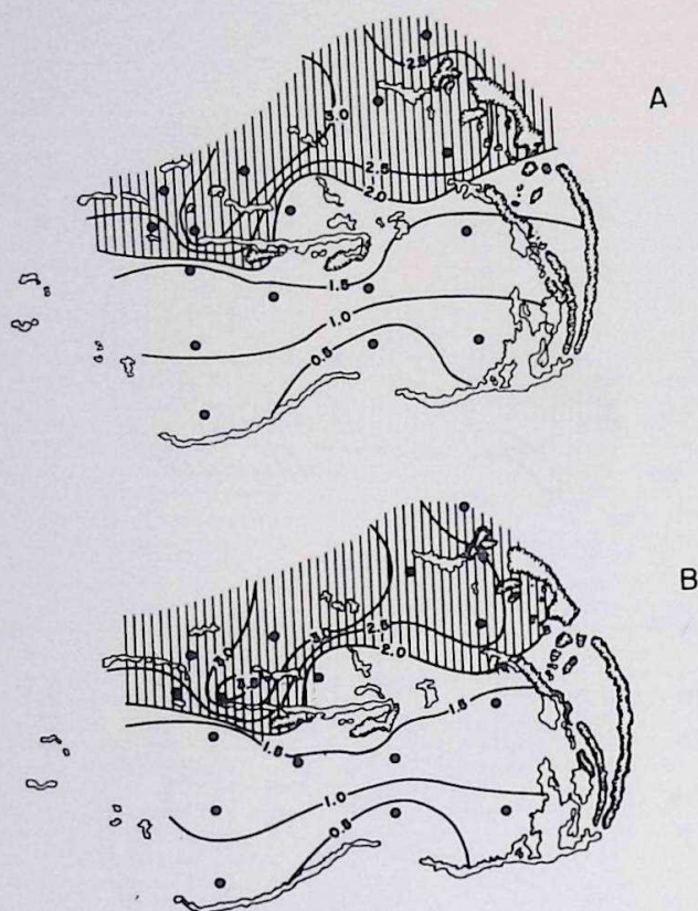
Figura 5.- Distribución horizontal (A y B) del contenido de fósforo orgánico (P-org. %) y fósforo total (P-total %) en los sedimentos del Archipiélago Los Roques.
