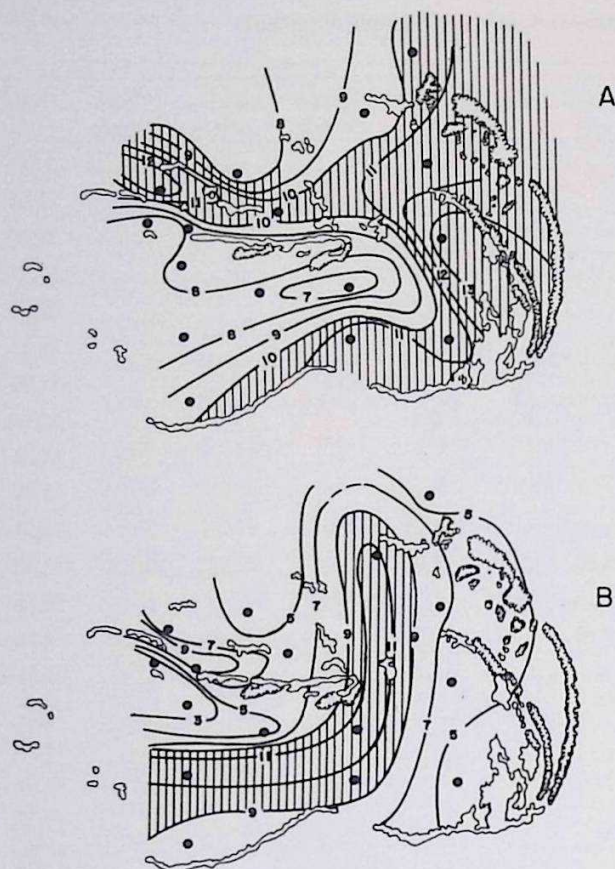
Figura 3.- Evolución horizontal (A y B) del valor de la Razón C/N y de la materia orgánica total (MOT) en los sedimentos del Archipiélago Los Roques.
