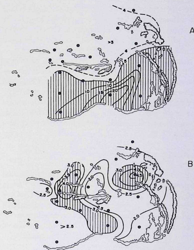
Figura 6.- Evolución espacial (A y B) de las razones N/P y el contenido de carbohidrato totales (CHT mg/g) en los sedimentos del Archipiélago Los Roques.
